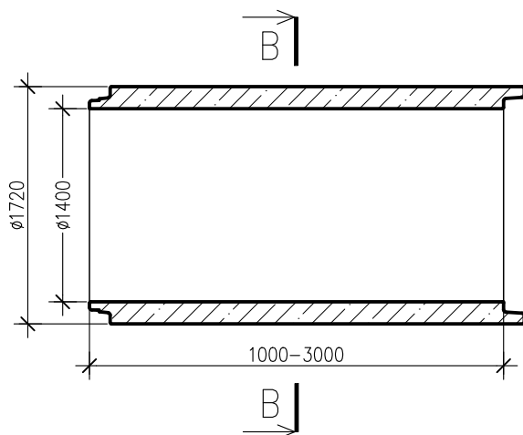
PRZEKRÓJ A-A
